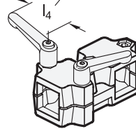
Ayarlanabilir el manivelası GN 911
